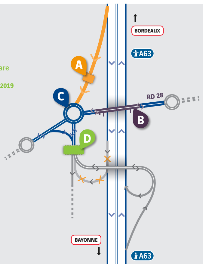
Le nouveau pont de la RD 28
